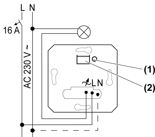
Bild 1: Anschlussplan
