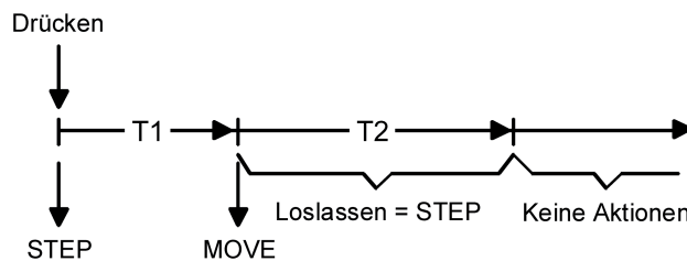
Bild 21: Bedienkonzept "Kurz-Lang-Kurz"
