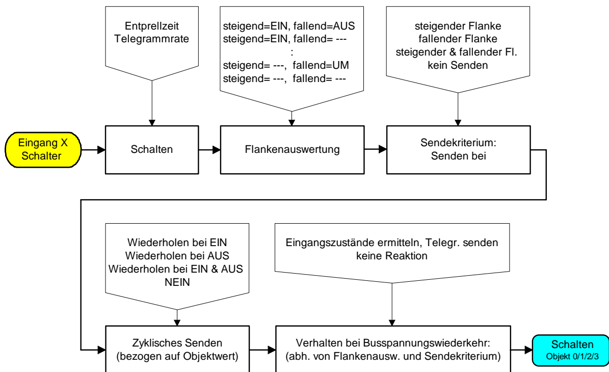
Funktionsschaltbild
